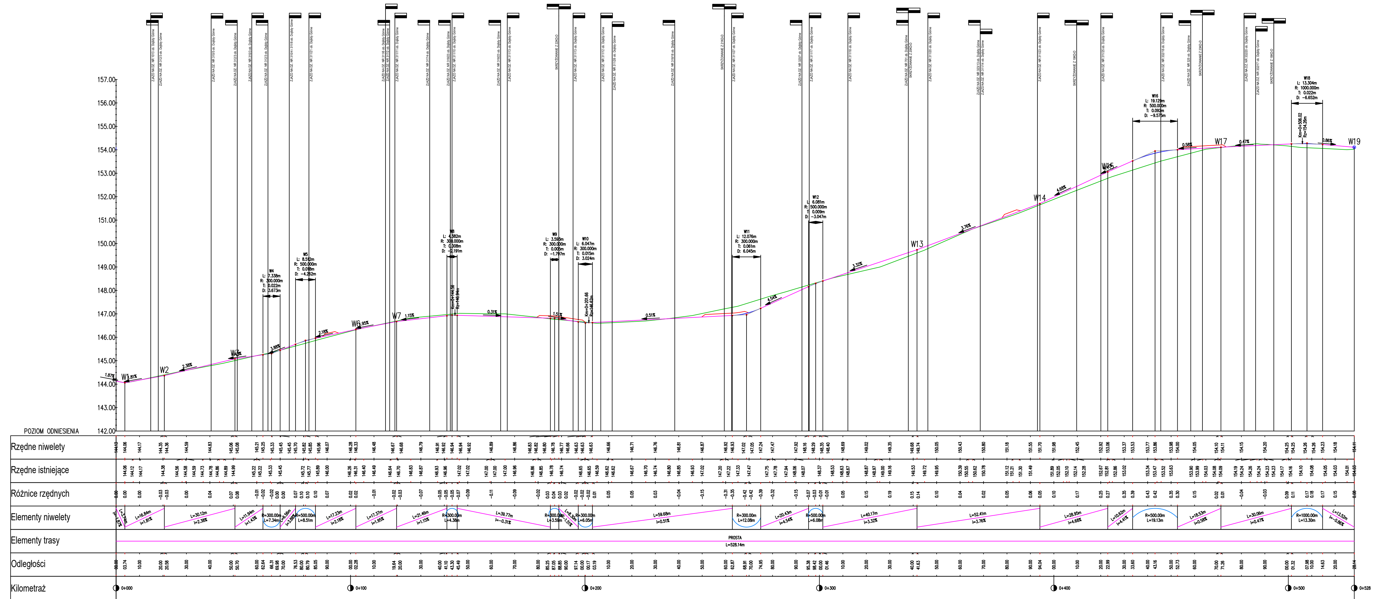
Profil podłużny - ul. Motyla 7KD-D
