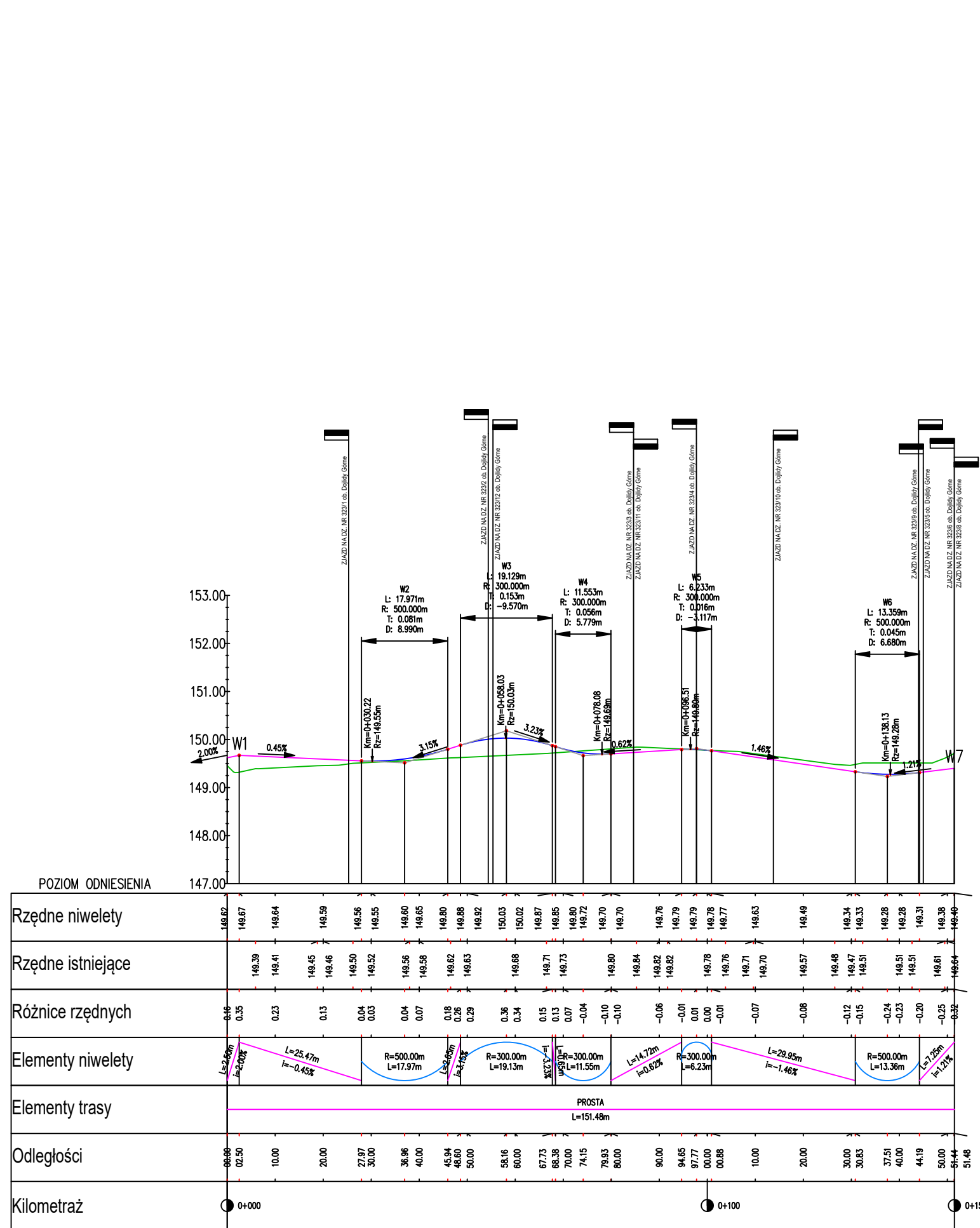
Profil podłużny - sięgacz 20KD-D
